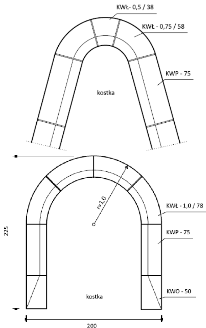
Rysunek 1 –Przykładowy krawężnik wyspowy z narożnikiem łukowym
