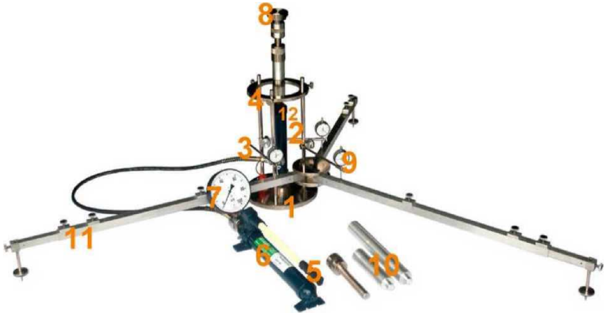
Rys. 1.2. Aparatura VSS z jednopunktowym pomiarem przemieszczenia płyty
