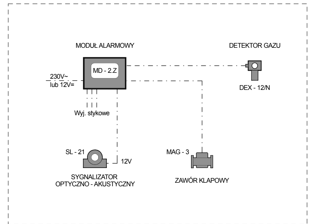
SCHEMAT BLOKOWY ASBIG
